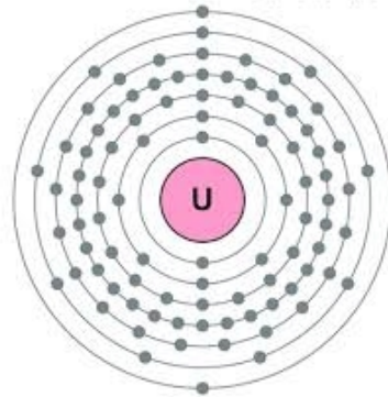
92: Uranium
