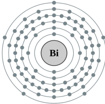
83: Bismuth
