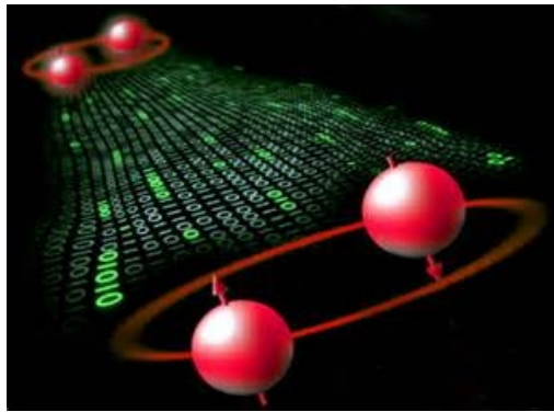
Quantum entanglement
